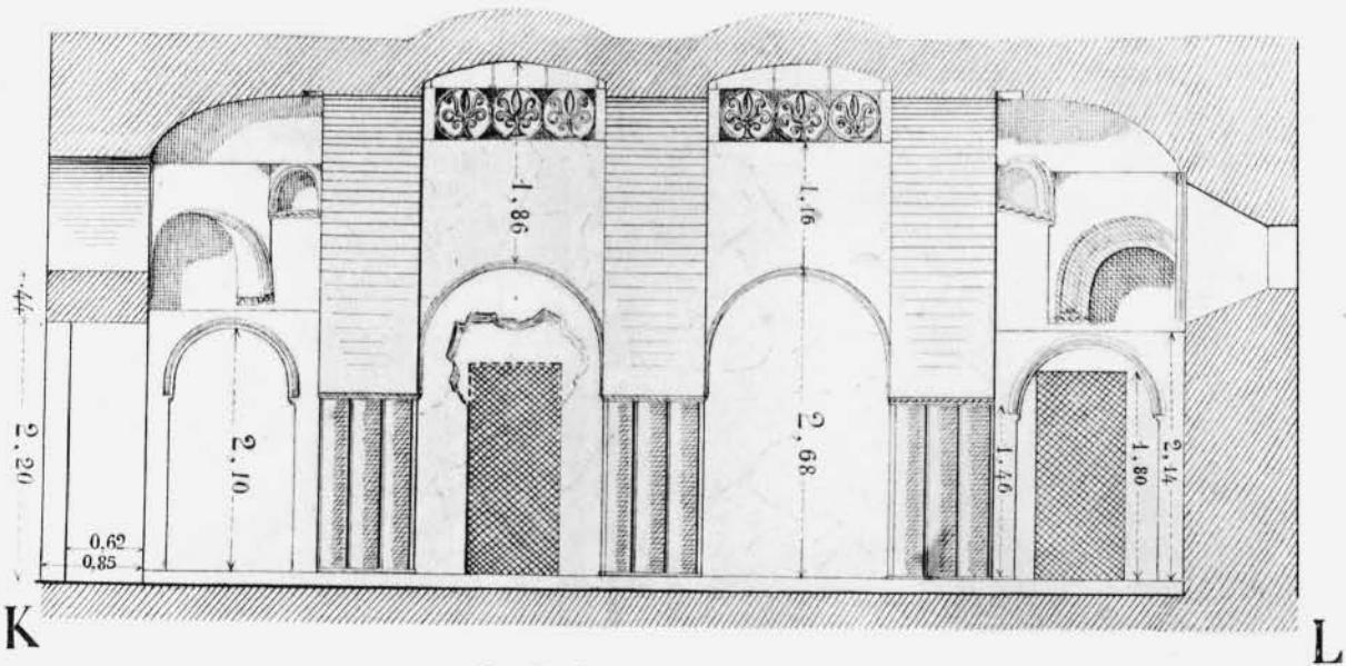
QASR-HARÂNEH. - Plan et coupe de la salle 51.
