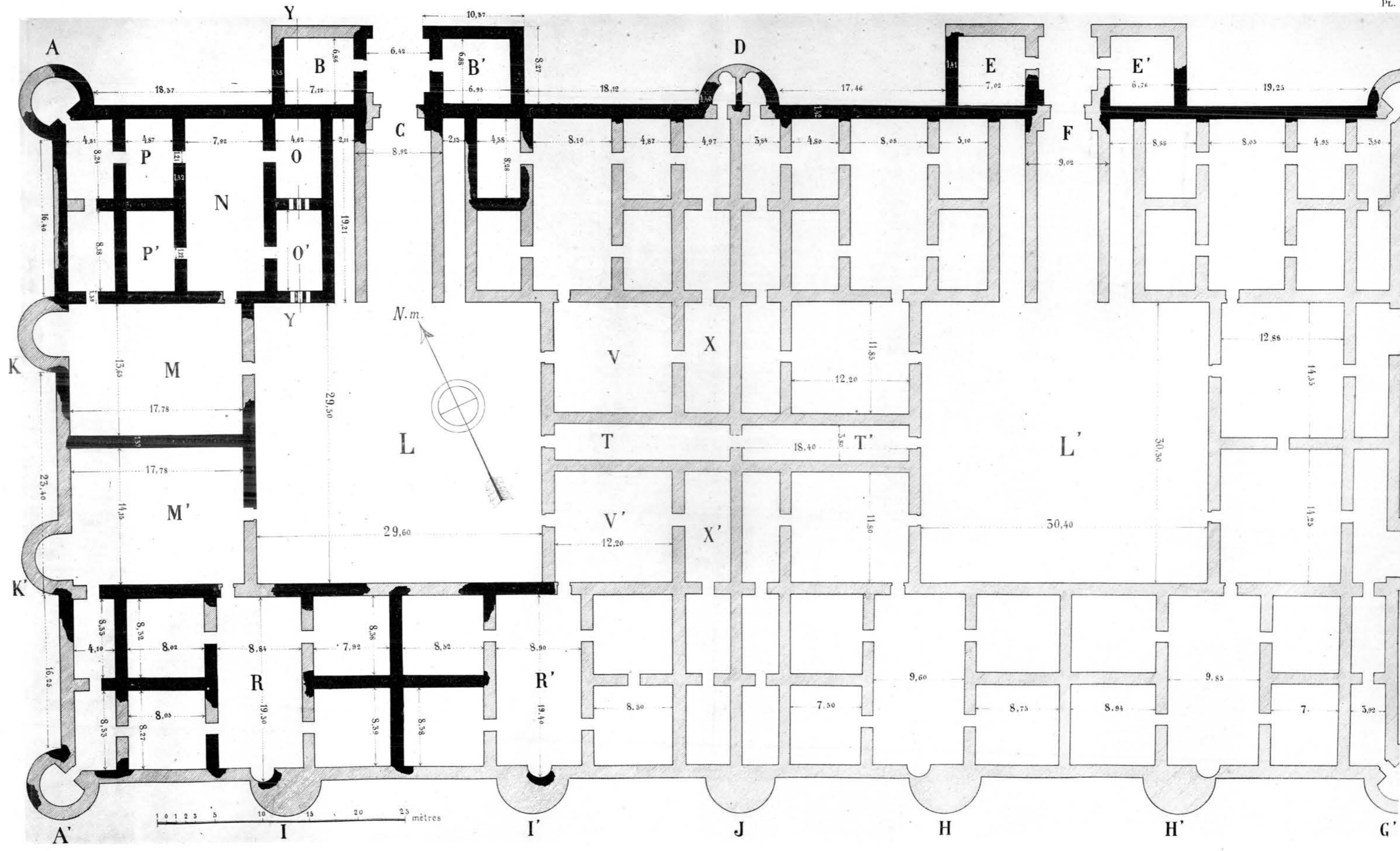
QASR ET-TÛBA. — Plan général des ruines.
