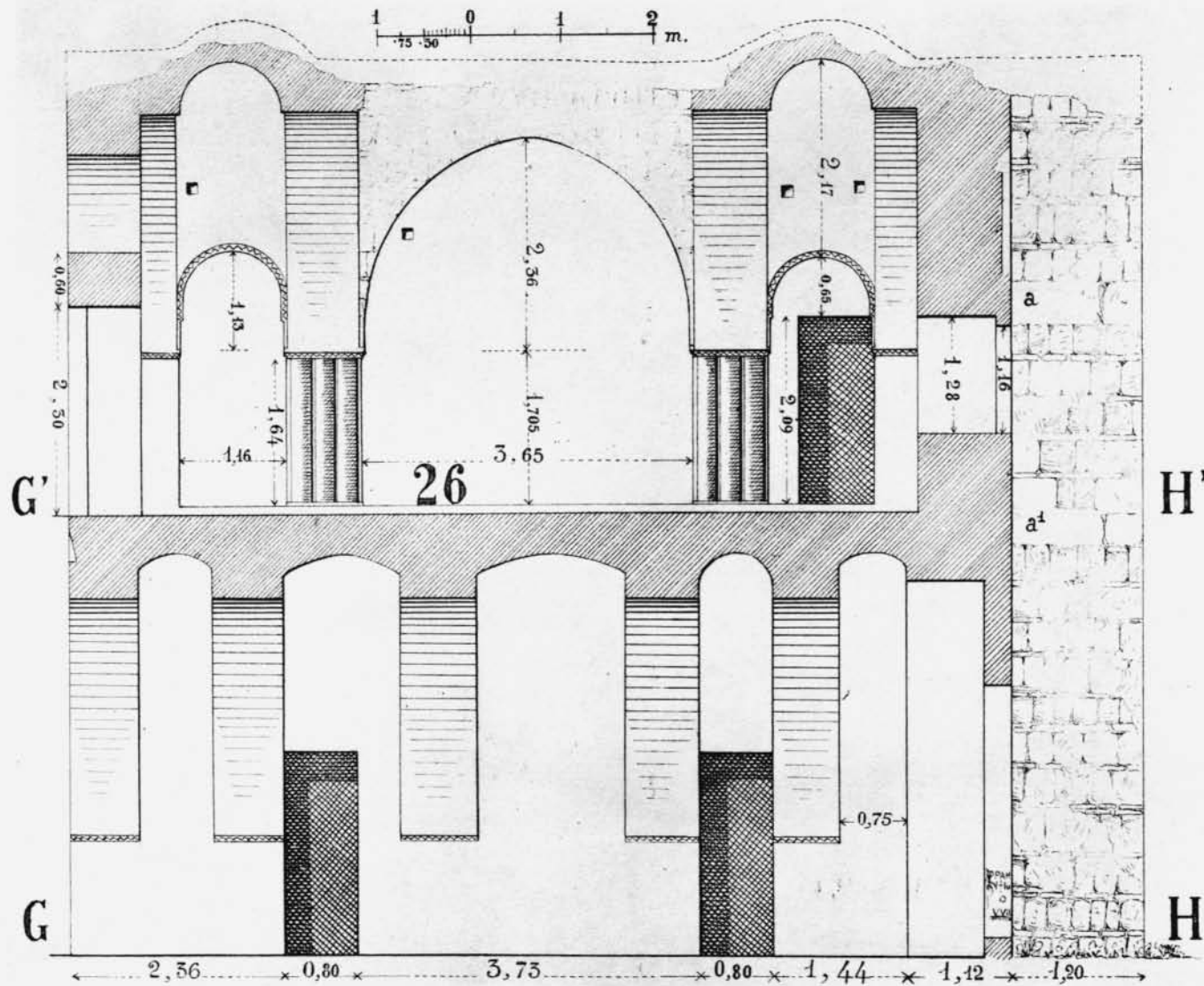
QASR-HARÂNEH. - Coupes longitudinales du corridor d'entrée du rez-de-chaussée et de la salle 26 à l'étage supérieur. - (Voir le plan par terre, pl. XXIII et le plan de l'étage, pl. XXIV, avec la figure 11.)
