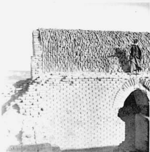
2. — QASR ET-TÛBA. — Reste d'absidiole à l'intérieur de la tour D.
