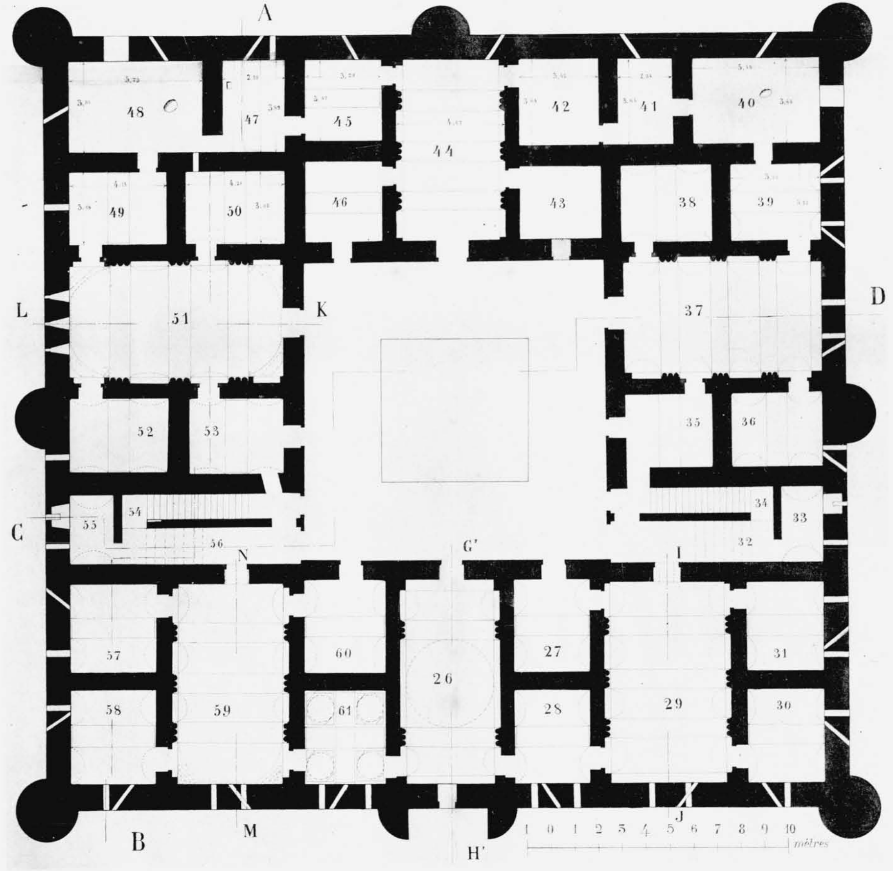
QASR-HARÂNEH. - Plan de l'étage.
