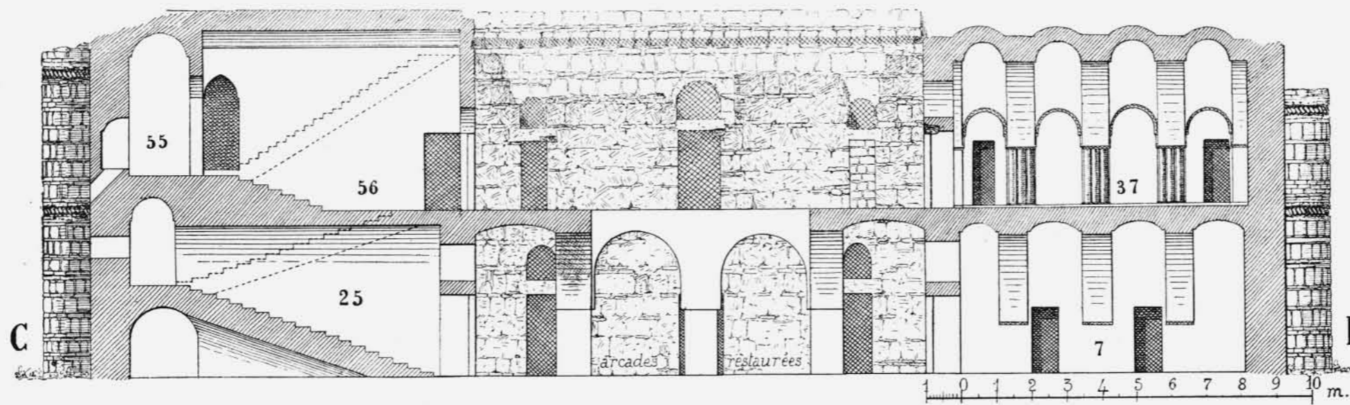
QASR HARANEH. — Coupes sur AB et CD. (Voir les Plans, pl. XXIII et XXIV.)
