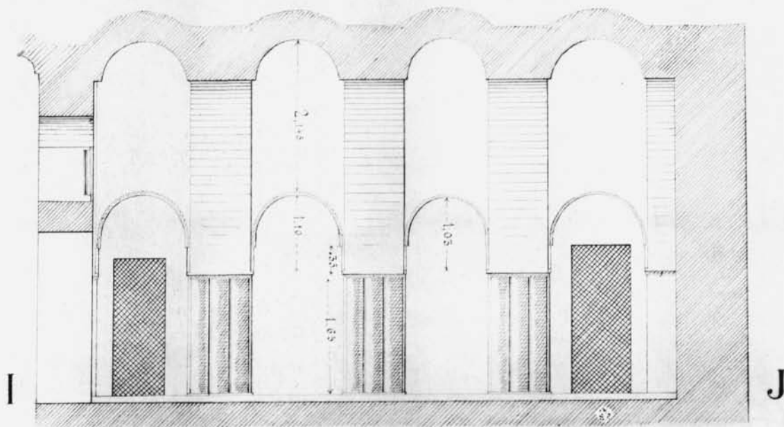
QASR-HARÂNEH. - Plan et coupe de la salle 29.
