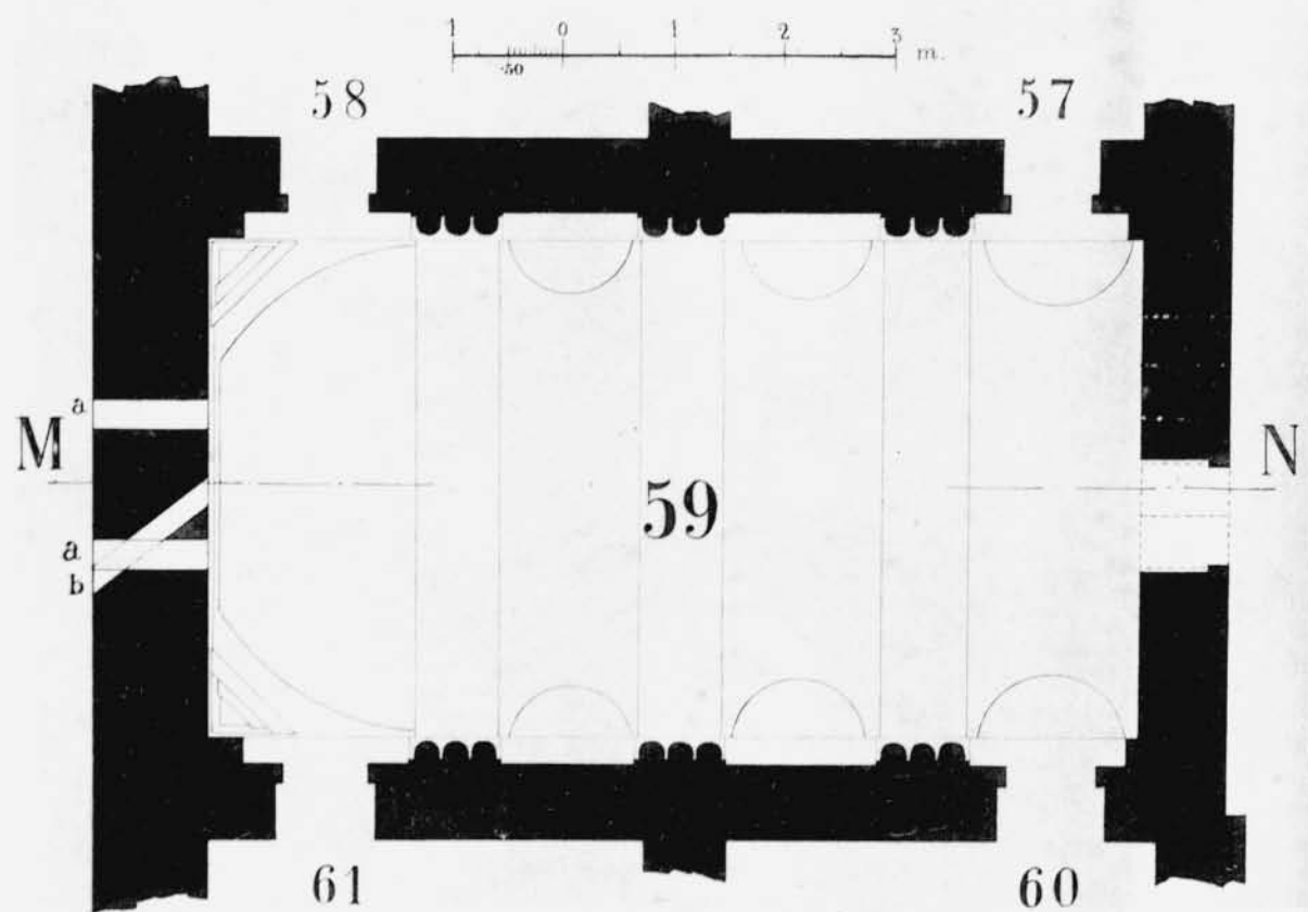
QAŞR-HARÂNEH. - Plan et coupe de la salle 59.
