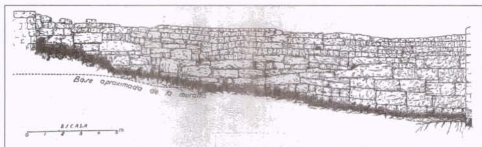
FIGURA 1 ALÇAT DEL SECTOR LLEVANTÍ DE LA MURALLA DEL RECINTE FORTIFICAT DE SANT MIQUEL D'OLÈRDOLA
