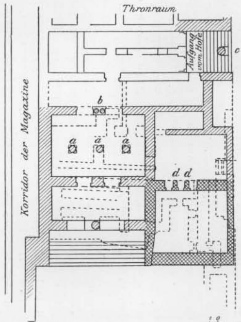
Knossos, Obergeschoß nach Evans' Rekonstruktion.
