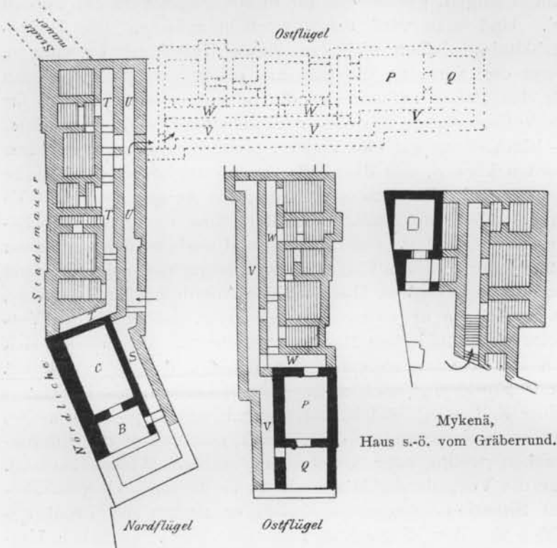
Palast von Arne (die wirkliche Lage des Ostflügels ist durch punktierte Linien angegeben)
