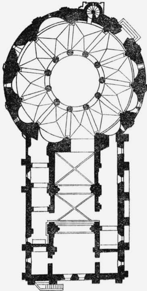
FIG. 1. — Église de Neuvy-Saint-Sépulcre (Indre). Plan. (Monuments historiques)
