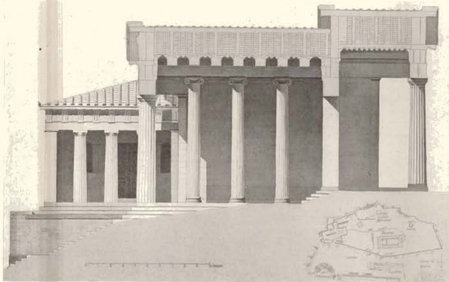
Les Propylées de l'Acropole d'Athènes. Coupe longitudinale restituée par E. Ullmann (D'après d'Espouy. Fragments antiques . Massin, éditeur).
