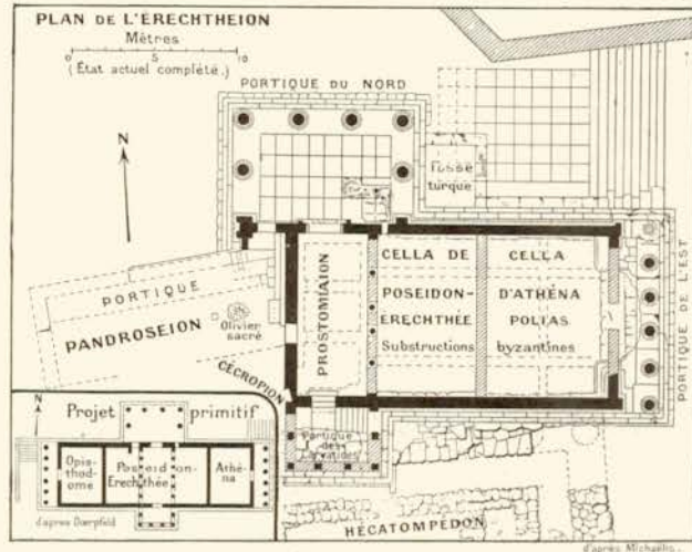
Plan et projet primitif de l'Erechtheion.
