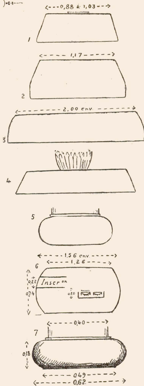
Fig. 13. — Bases préhelléniques : 1-3. Mishrifé (Qatna) vers 2300. — 4. Égypte (XVIII e -XIX e dynasties), cf. PERROT et CHUPIEZ, I, p. 565, fig. 345 (Toutmès III) et p. 567, fig. 346 (Ramesseum). — 5. Assyrie (Khorsabad). — 6. Tell el-Yahoudiyé (Ramsès III). — 7. Base de colonne en basalte à Tell Nebi Mend.
