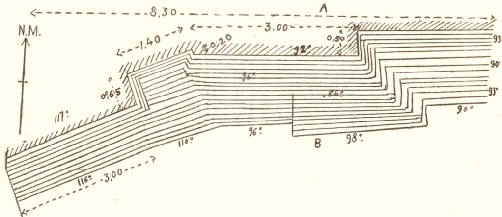
Fig. 4. — Plan du mur de briques crues couvrant les levées de sable du Nord (parement du Sud).
