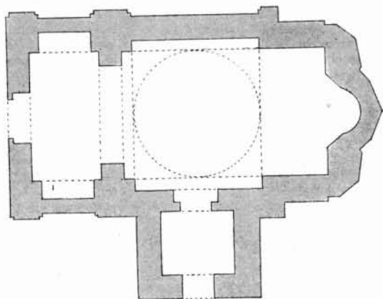
FIG. 87. — Kuršumlija. Plan au \frac{1}{200} .
