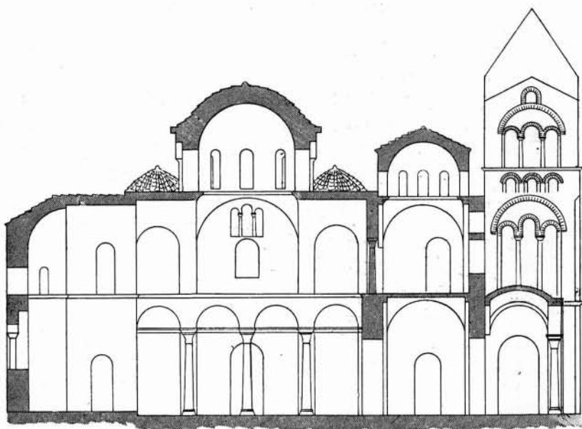
FIG. 49. — Église du Brontochion à Mistra. Coupe longitudinale d'après les Monuments byz. de Mistra .
