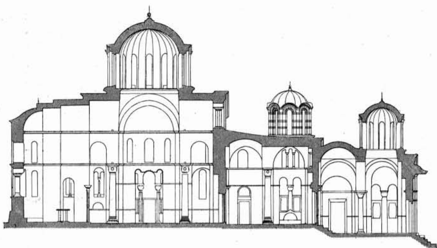
FIG. 28. — Église de Chilandari au Mont-Athos. Coupe longitudinale.
