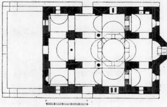
FIG. 141. — Église de Gastouni en Élide.
