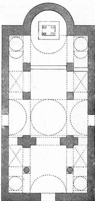
FIG. 46. — Nagoriča. Plan au \frac{1}{200} .
