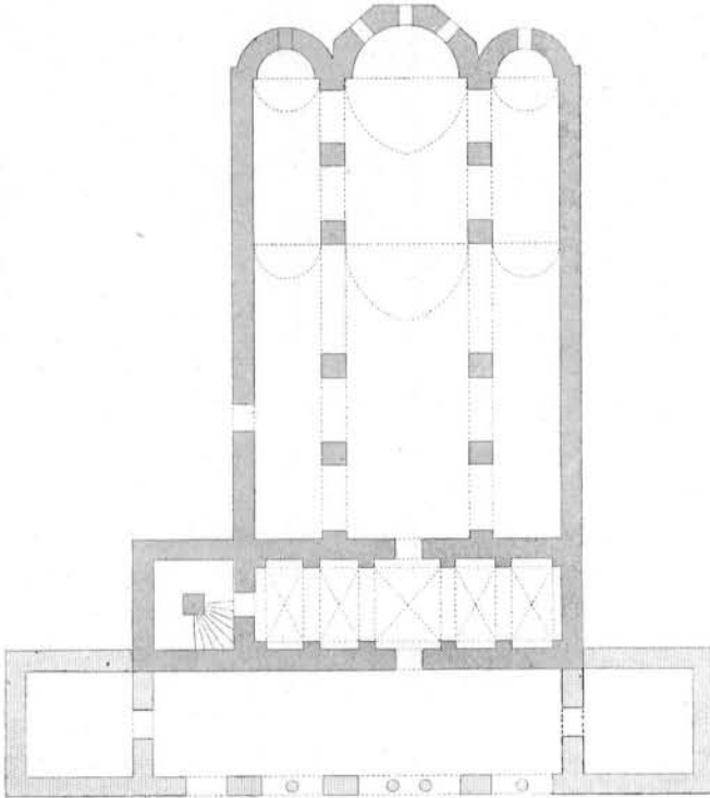
FIG. 19. — Sainte-Sophie d'Ochrida. Plan au \frac{1}{400} .
