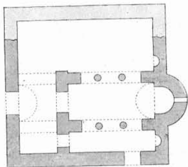
FIG. 9. — Basilique des Taxiarches. Plan au \frac{1}{200} .
