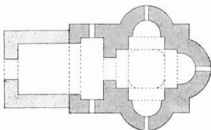
FIG. 48. — Coubelitissa, Plan au \frac{1}{200} .
