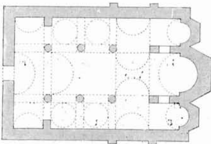
FIG. 24. — Kato-Panaghia. Plan d'après Lampakis (rectifié).
