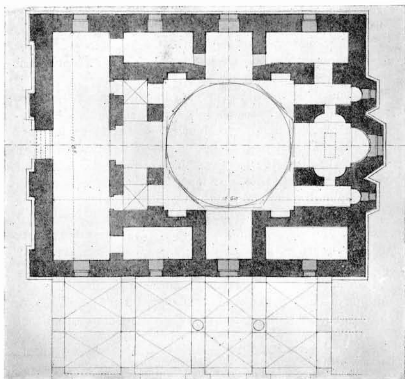
FIG. 59-60. — Église de Sainte-Sophie à Monemvasie. Plan et coupe longitudinale. Dessins de L. Chesnay, propriété des Monuments Historiques, au \frac{1}{200} 8
