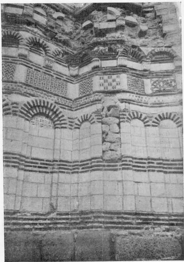
FIG. 123. — Église de Saint-Jean-Alitourgitos à Mésemvrie. Détail des absides.
