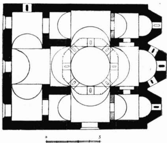
FIG. 144. — Église de Saint-Théodore à Athènes.
