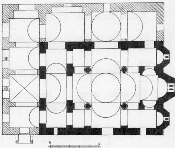
FIG. 145. — Église de la Capnicaréa à Athènes.
