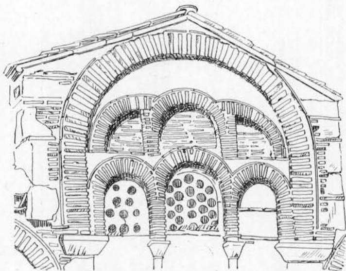
FIG. 104. — Catholicon de Saint-Luc. Fenêtre, sur la façade Sud.
