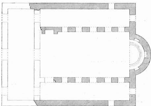
FIG. 4. — Basilique de Mésenvrie. Plan au \frac{1}{400} .
