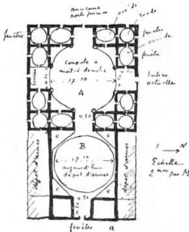
FIG. 55. Église des Nestoriens à Amida. Relevé du général de Beylié, d'après Berchem-Strzygowski.
