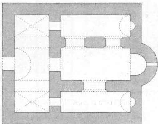
FIG. 7. — Basilique des Saints-Anargyres. Plan au \frac{1}{200} .
