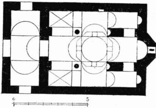
FIG. 139. — Église de Saint-Jean à Koroni (Argolide).
