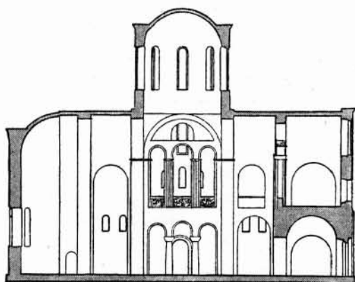
FIG. 50. — Église du Sauveur à Černigov. Coupe longitudinale d'après Pavlinov.
