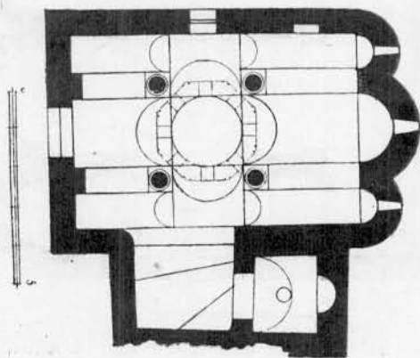
FIG. 146. — Église de la Transfiguration, au Nord de l'Acropole.
