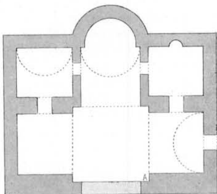
FIG. 33. — Souldjé-Djami à Salonique. Plan au \frac{1}{200} .
