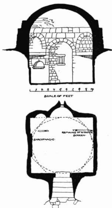
FIG. 54. — Église du Sauveur à Milo. Plan et coupe d'après Fletcher-Kitson.
