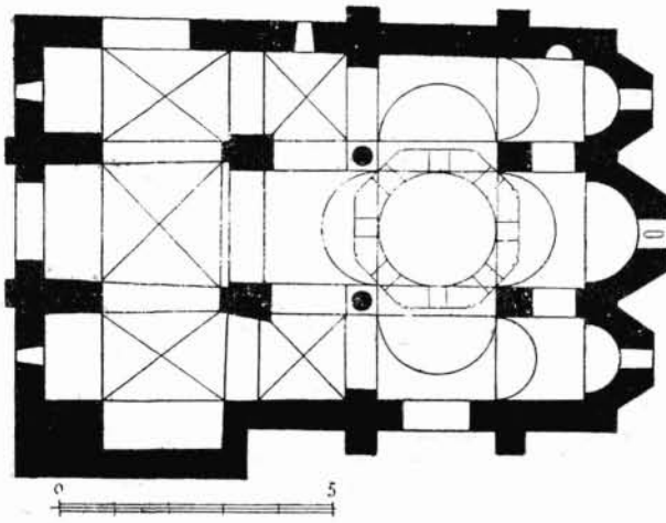
FIG. 140. — Église du Sauveur à Amphissa.
