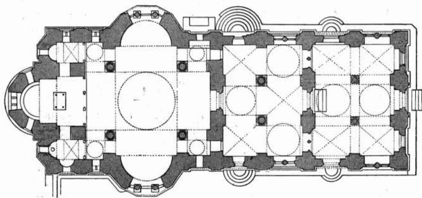
FIG. 29. — Chilandari. Plan. Dessins de la Mission Sévastianov.
