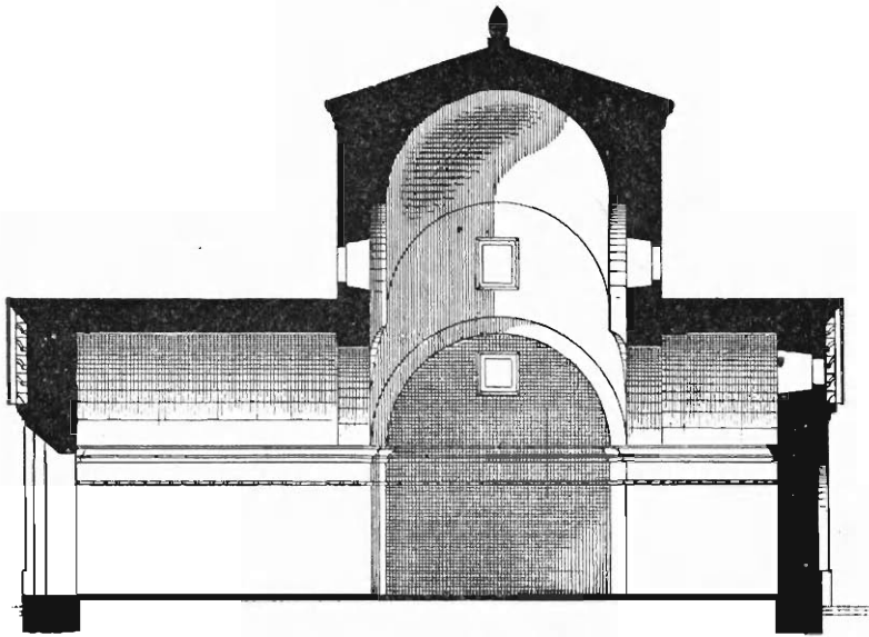
Fig. 2. Längenschnitt.
