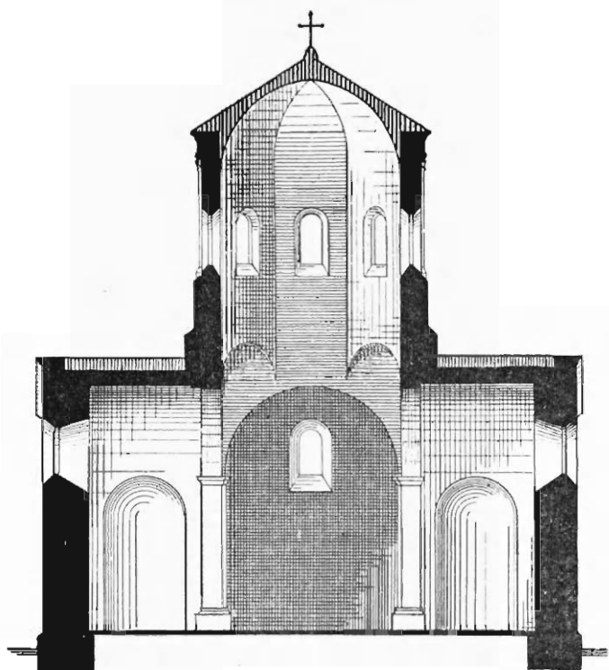
Fig. 5. Querschnitt
