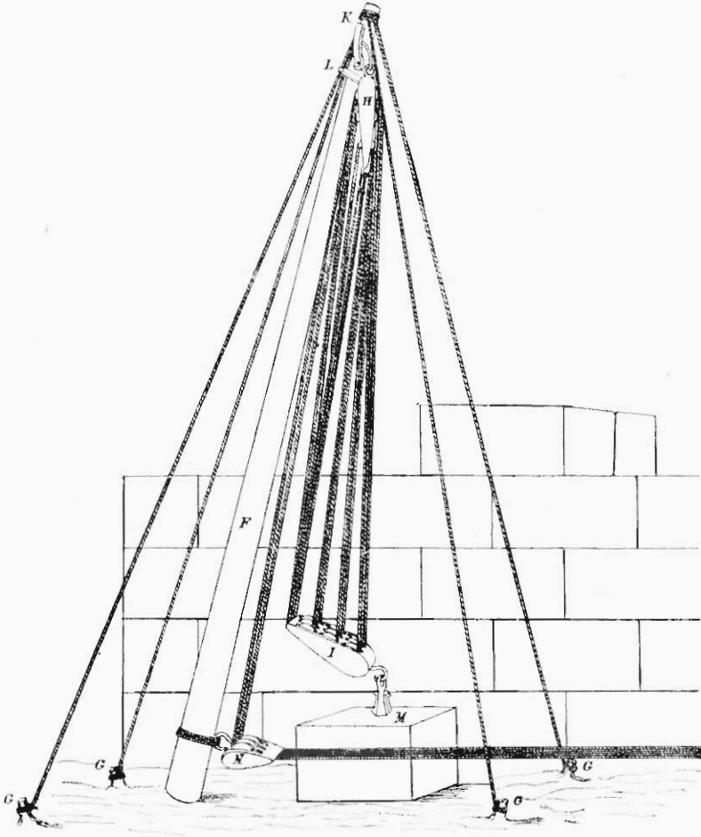
Fig. 18. — Polyspaste.
