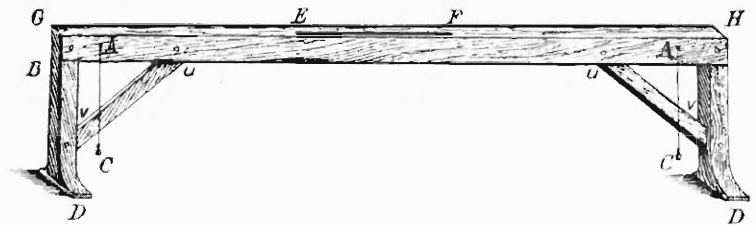
Fig. 13. — Le chorobate. Restitution de Newton.
