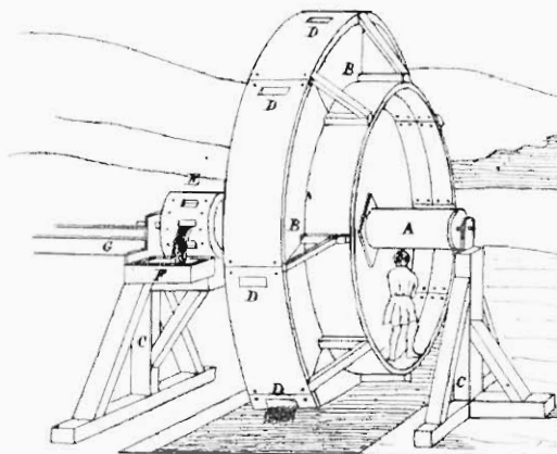
Fig. 21. — Tympan à élever l'eau.
