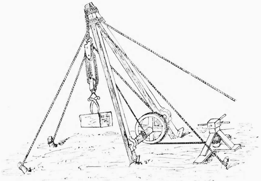
Fig. 16. — Trispaste double (d'après Blümner).
