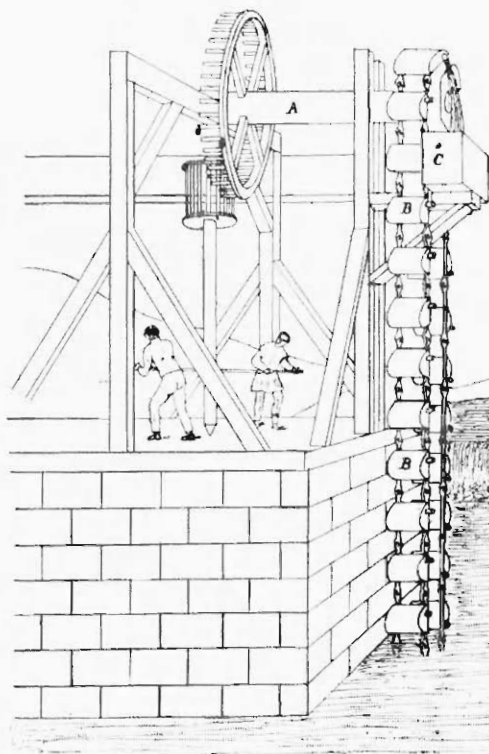
Fig. 23. — La noria, d'après Vitruve.
