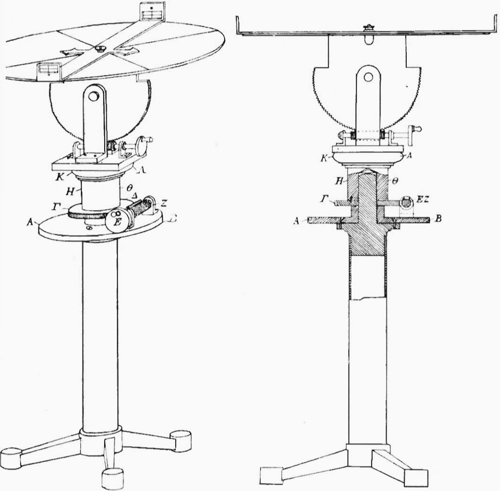
Fig. 5. — Dioptra de Héron, restituée par Schœne.
