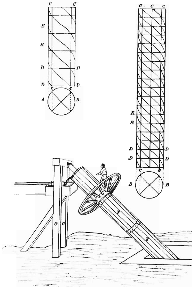
Fig. 20. — Vis d'Archimède.
