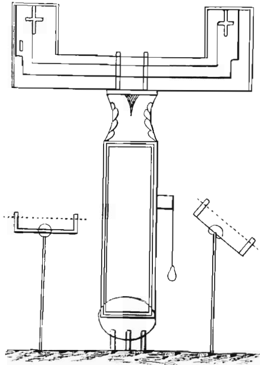
Fig. 3. — Dioptré de Héron. Dessin du manuscrit.
