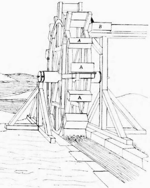
Fig. 22. — Roue à aubes planes et godets. pour élever l'eau d'une rivière.
