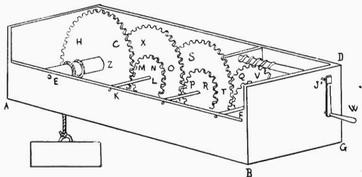
Fig. 19. — Appareil de traction et d'élévation (βαρούλκος) de Héron.
